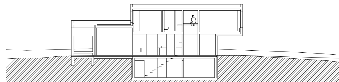
Schnitt
